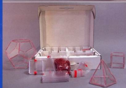
Basissatz es02 , bestehend aus: 40 gleichseitige Dreiecke, 30 Quadrate, 12 Fünfecke, 24 gleichschenklige Dreiecke, 20 Rechtecke, ca. 400 Gummiringe
