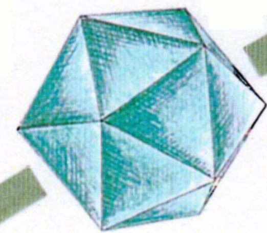
Ikosaeder
