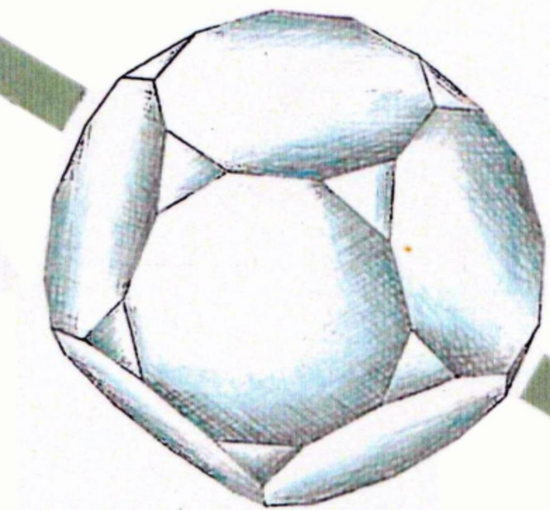
Dodekaederstumpf
