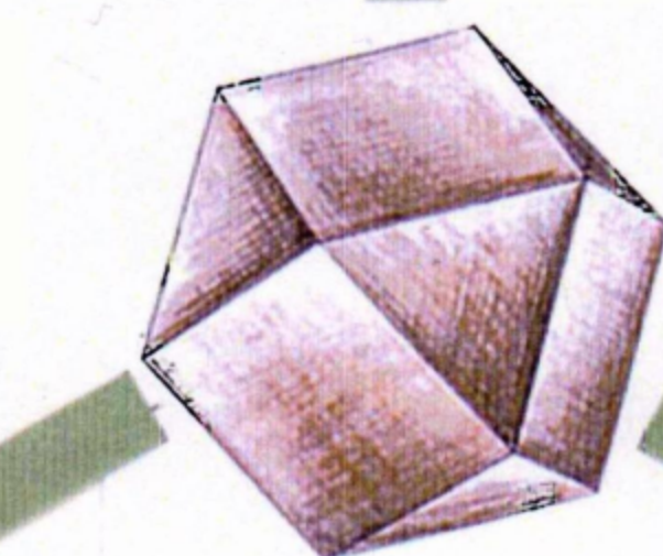
Kuboktaeder
