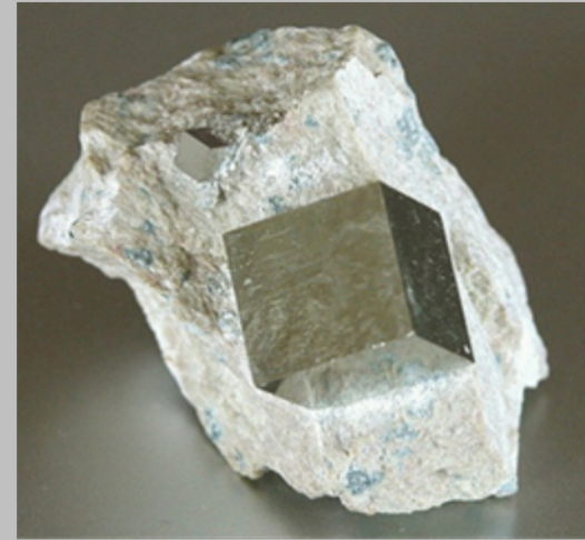
Pyrit
