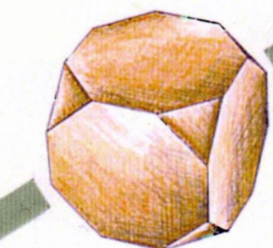
Würfelstumpf
