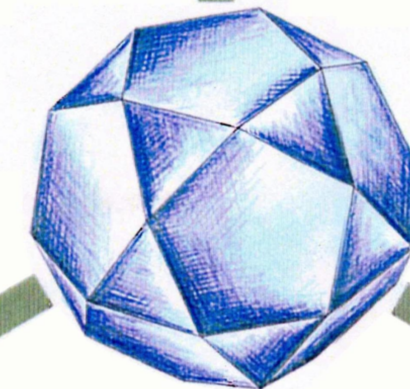
Ikositodekaeder
