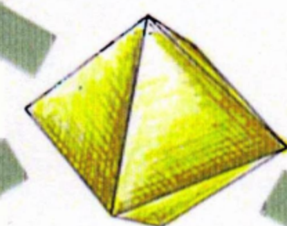
Oktaeder
