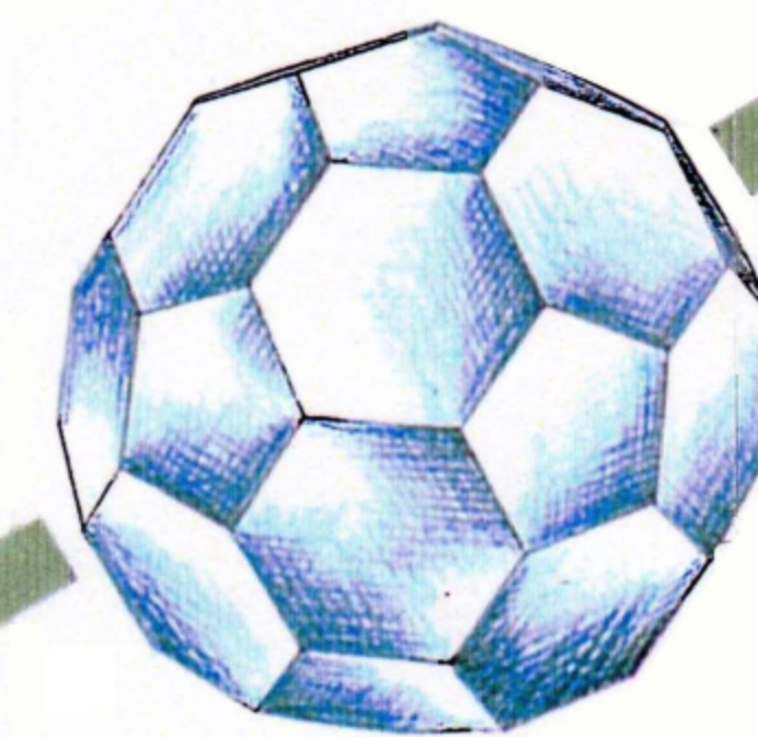
Ikosaederstumpf
