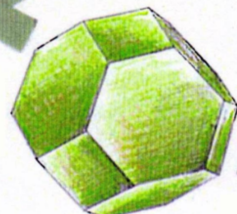
Oktaederstumpf
