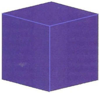
Würfel
